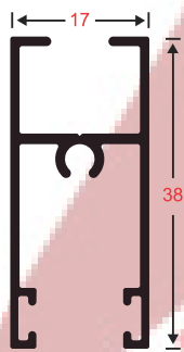
2004 CABEZAL
