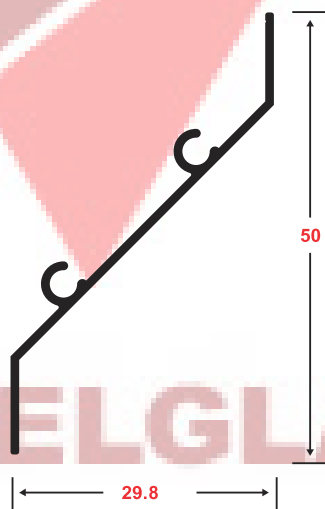
PERFIL PERSIANA
