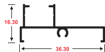
2629 MARCO FIJO
