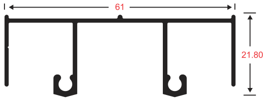
2004 CABEZAL
