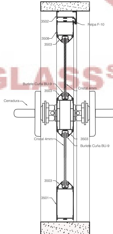
PUERTA BATIENTE VISTA VERTICAL
