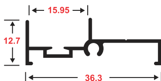
2628 MARCO MOVIL
