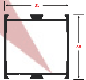
3508 Bastidor
