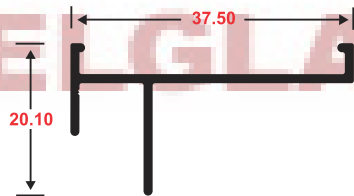
2626 RIEL SUPERIOR
