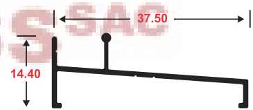
2627 RIEL INFERIOR
