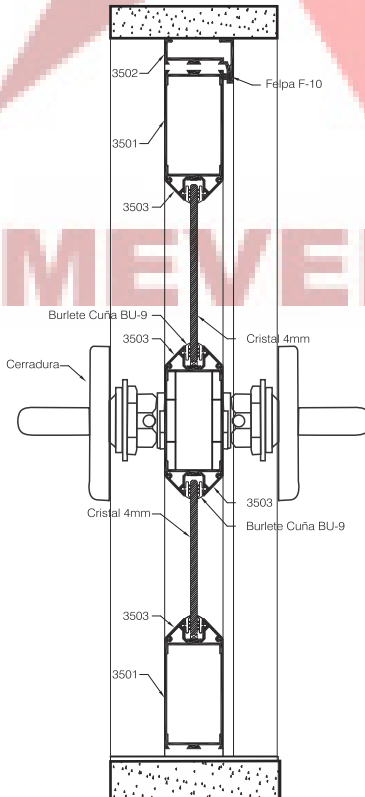
PUERTA BATIENTE VISTA VERTICAL
