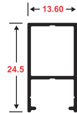
2624 HORIZONTAL MOVIL
