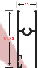
2627 RIEL INFERIOR
