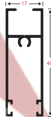
2005 ZÓCALO
